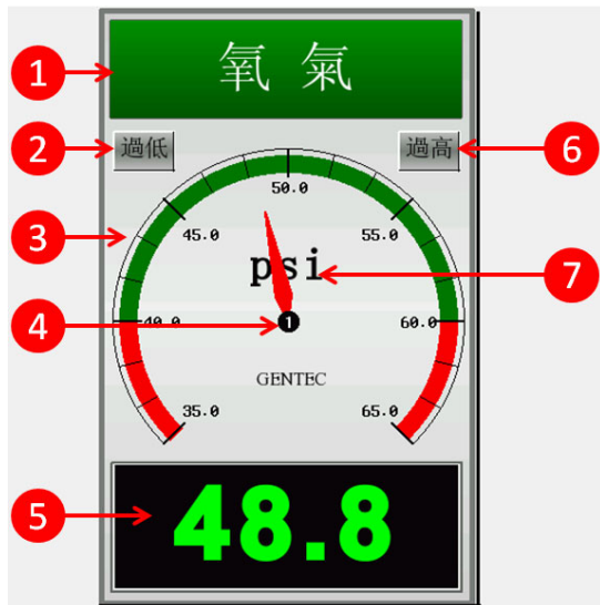
四氣以下壓力顯示錶
